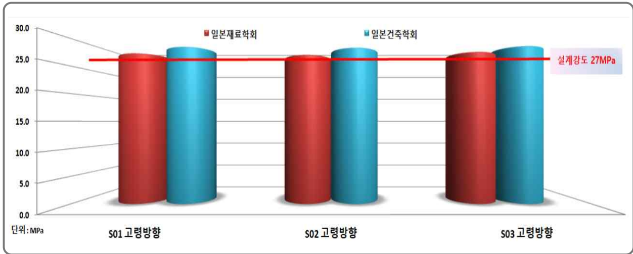
[그림 4.2.1] 반발경도법에 의한 비파괴강도 측정 결과-상부구조(바닥판하면)
